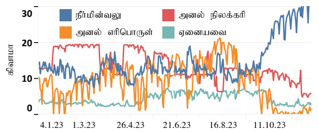
மூலங்கள் ரீதியான மின்வலு உருவாக்கம்
